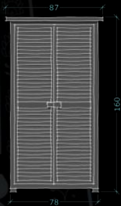
Vista Frontale
